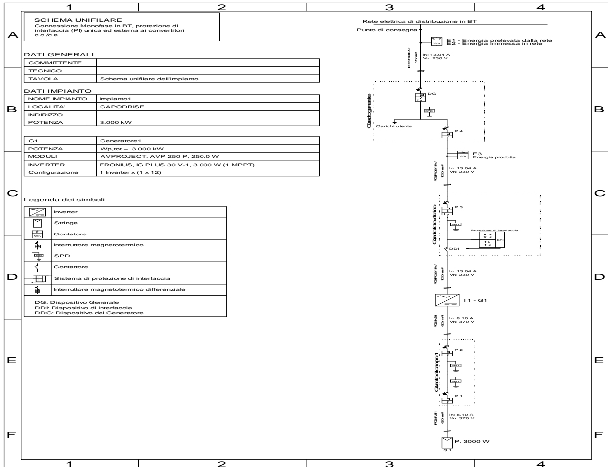
Fig. 6: Schema elettrico unifilare dell'impianto
